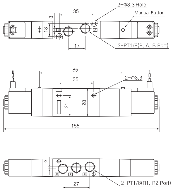
3position / 5port double (Grommet type)
