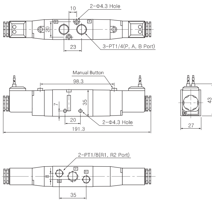
3position / 5port double(Lamp type)
